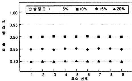
그림 9. 학습한 손상의 예측
