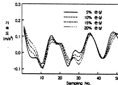
그림 8. 요소 2 손상시 가속도 응답
