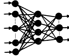
그림 2. 다층퍼셉트론
