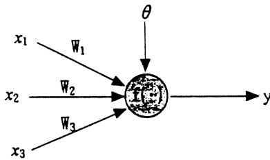
그림 1. 인공신경망의 뉴우런
