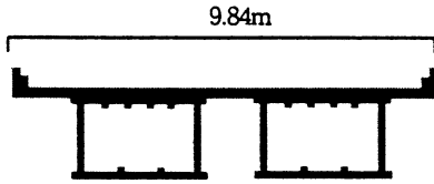
(b) 강박스거더교의 횡단면
