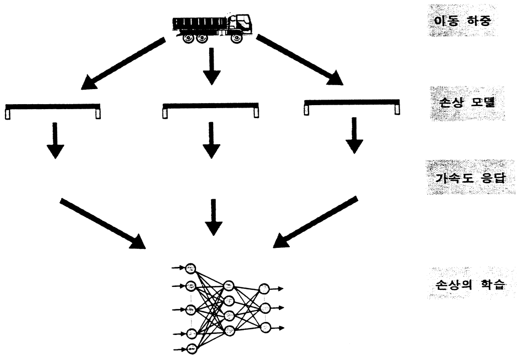
그림 3. 손상평가를 위한 신경망 학습 개념도
