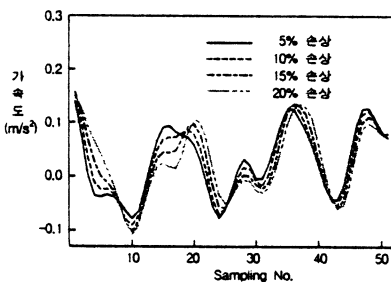
그림 7. 요소 1 손상시 가속도 응답
