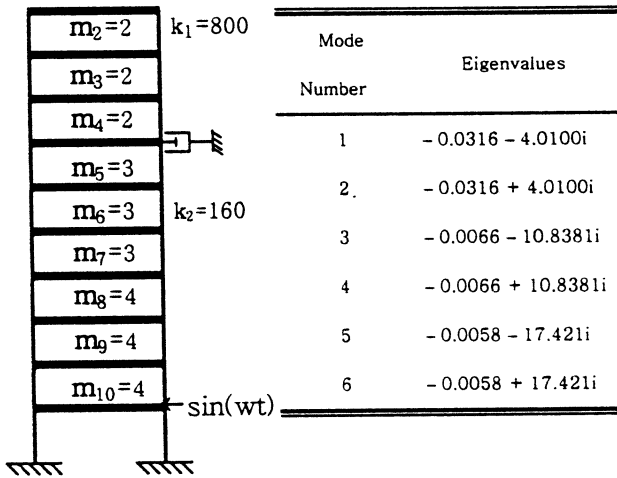
그림4 예제 구조물과 고유치
