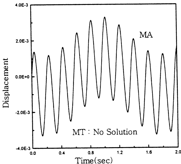
그림5 MA, MT방법의 응답 곡선
