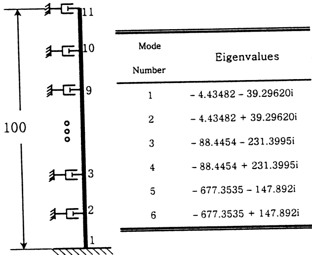
그림 1 예제 구조물과 고유치
