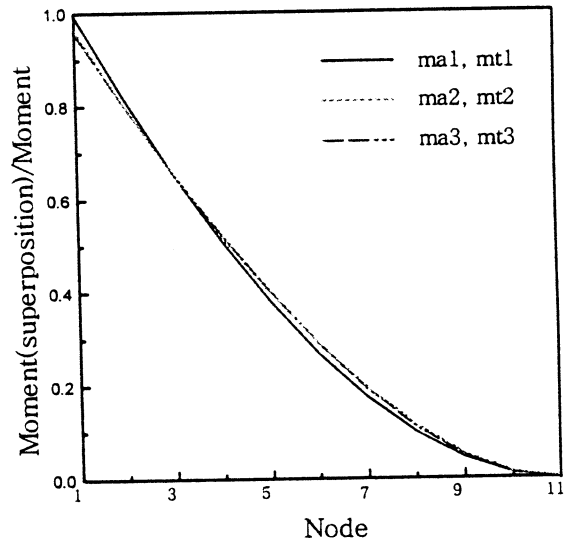
그림3 MA방법과 MT방법에 의한 모멘트
