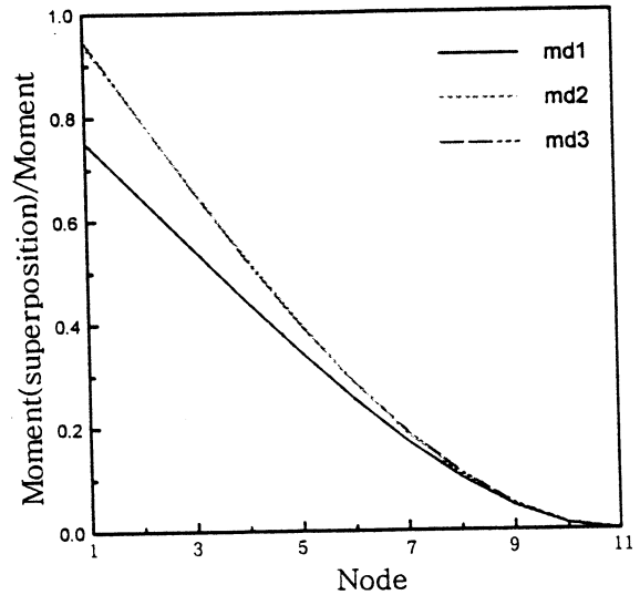
그림2 MD방법에 의한 모멘트
