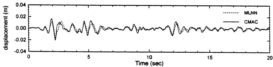
그림 3. 진동제어 결과 비교(El Centro, 3층의 변위)
