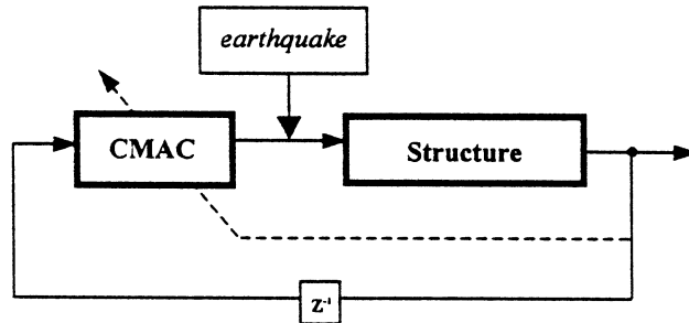
그림 1. 제어 블럭선도
