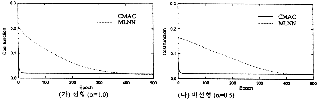
그림 2. 신경망의 학습 이력 비교
