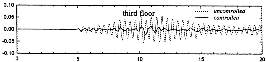
그림 4. Northridge 지진 시 3층의 변위 비교
