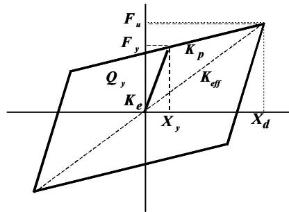
그림 1. 납고무 받침의 거동 및 설계 요소
