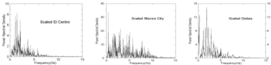
그림 4. 각 역사 지진의 Power Spectral Density
