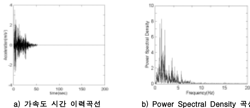
그림 3. 설계 지진 하중 (Scaled El Centro지진)
