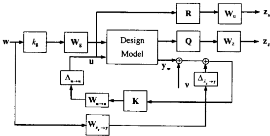
그림 2. 다양한 주파수 가중 필터를 포함한 \mu -제어기
