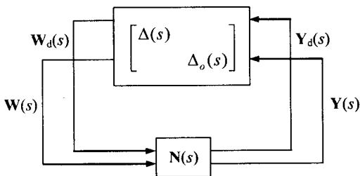
그림 1. 강인성 해석을 위한 표준형
