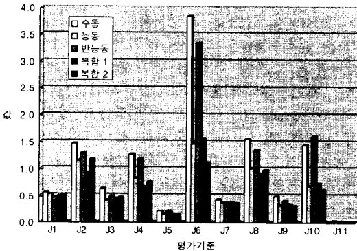
그림 3. 3 개의 지진에 대한 최대 평가기준
