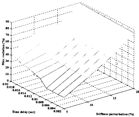
그림 4. 강성행렬의 불확실성과 유압식 가력기의 시간지연이 동시에 있을 때 강인성 (질량행렬의 불확실성이 없을 때)
