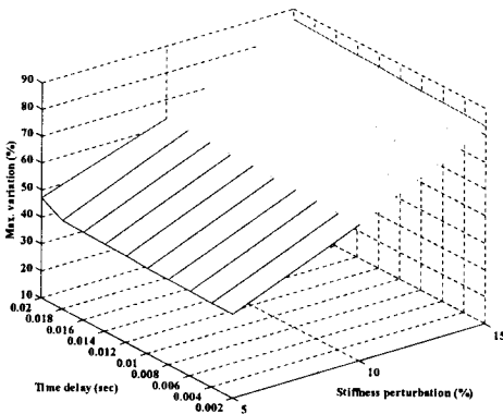
그림 4. 강성행렬의 불확실성과 유압식 가력기의 시간지연이 동시에 있을 때 강인성 (질량행렬의 불확실성이 있을 때)
