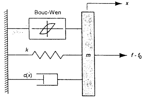
그림 4. MR 유체 감쇠기의 제안된 역학적 모델
