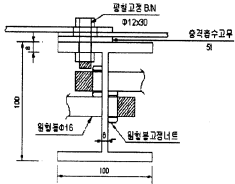
그림 8. H빔 지주 조립단면도
