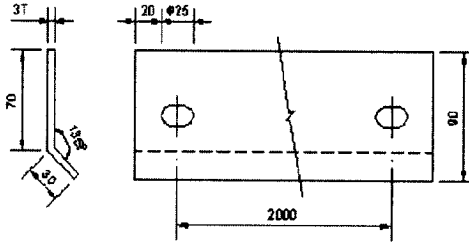
그림 5. L형 평철 상세도
