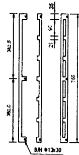
그림 6. 평철 보조대 상세도
