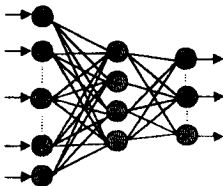
그림 2. 다층퍼셉트론
