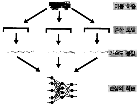
(그림 3) 손상평가를 위한 신경망 학습 개념도
