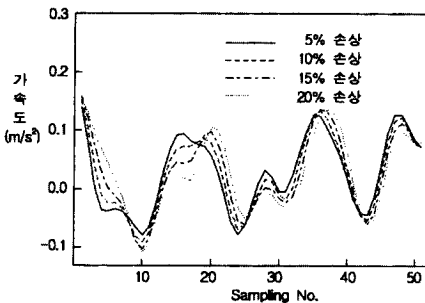
그림 7. 요소 1 손상시 가속도 응답
