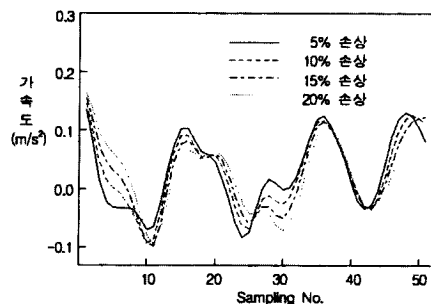
그림 8. 요소 2 손상시 가속도 응답
