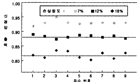
〈그림 10〉 학습하지 않은 손상의 예측
