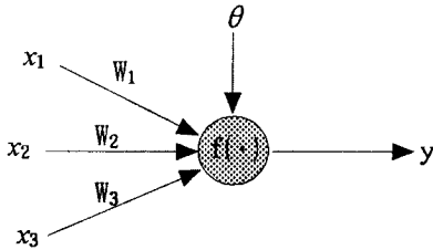
그림 1. 인공신경망의 뉴런
